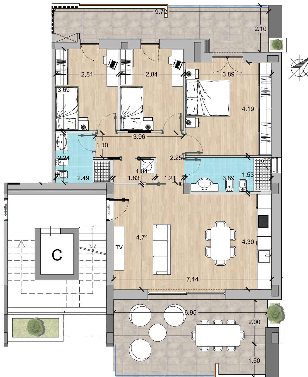
Pianta arredata - scala 1:100
