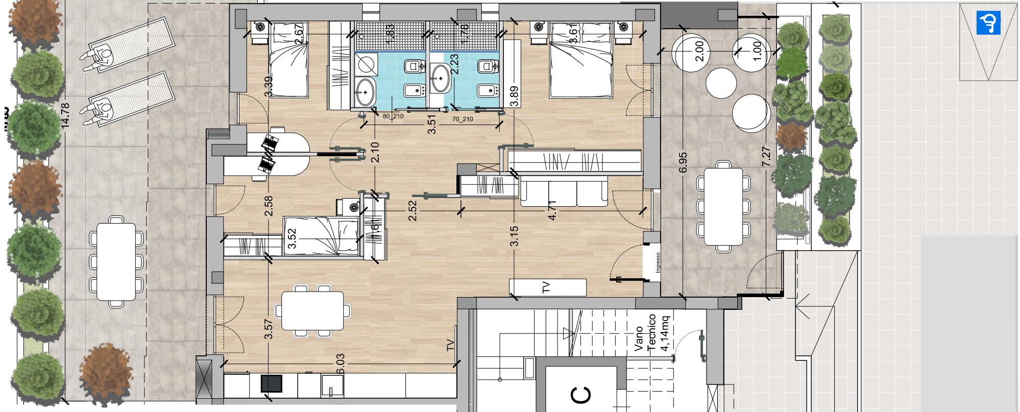
Pianta arredata - scala 1:100
