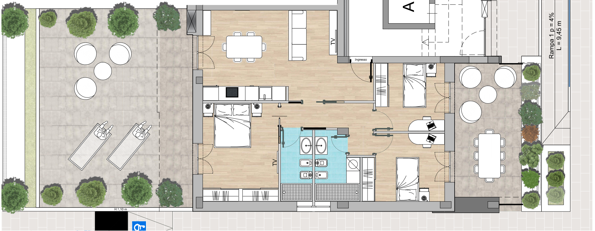
Pianta arredata - scala 1:100
